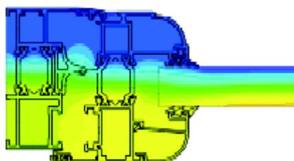
Diagrama de Isotermas
